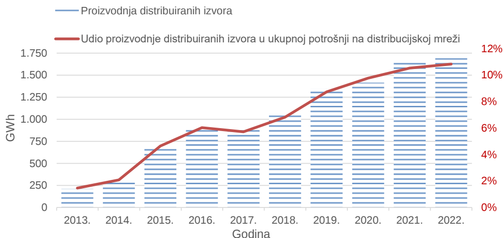
Slika 4.10 Godišnja proizvodnja električne energije iz distribuiranih izvora
